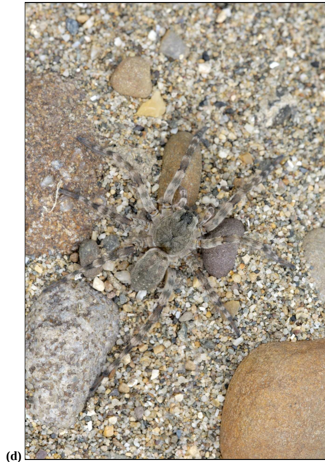
Figuur 3. De grindoevers (a) te Visserweert (NL) en (c) te Meers (NL), voorkeurs habitat respectievelijk voor (b) Pardosa agricola (Thorell, 1856) en (d) Arctosa cinerea (Fabricius, 1777). Foto's: a, c - K. Lambeets, 2005; b, d - R. Verlinde, 2007 (www.vildaphoto.net).
